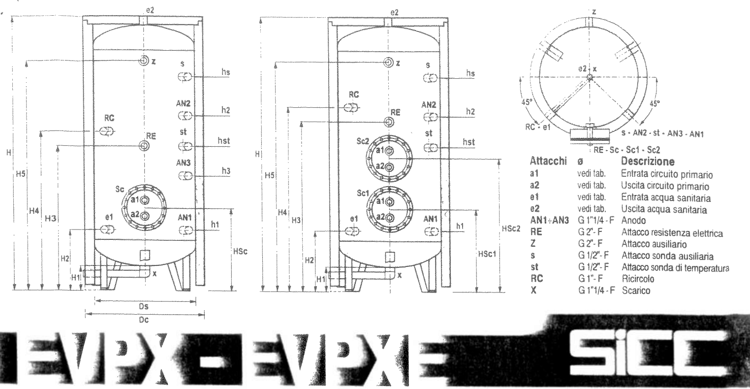
Dimensioni modelli a singolo scambiatore
